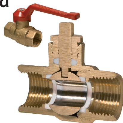
Przekrój zaworu kulowego Herz
