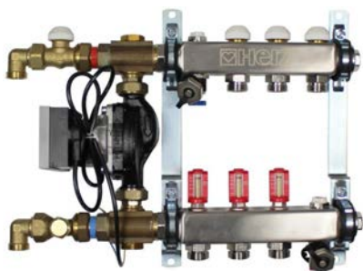
Fot. 1. Stacja rozdzielaczowa Compact Floor Light.
